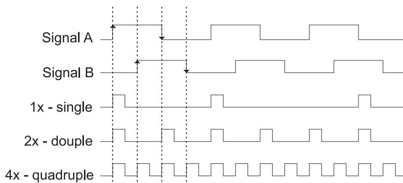
Figure 3-5 : Encoder inputs
