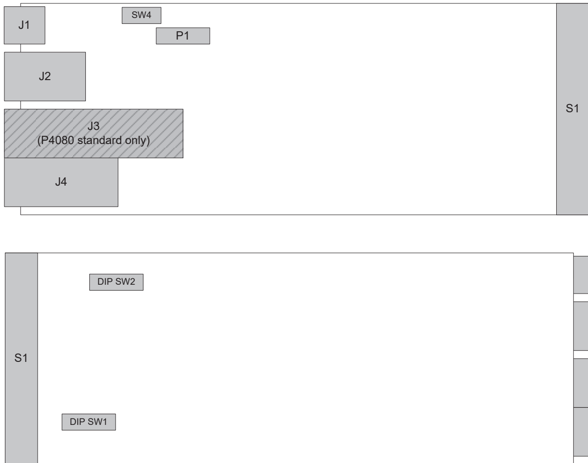
Figure 12: NAMC-QorIQ-Pxxx – Connector und Switch Location – Overview
